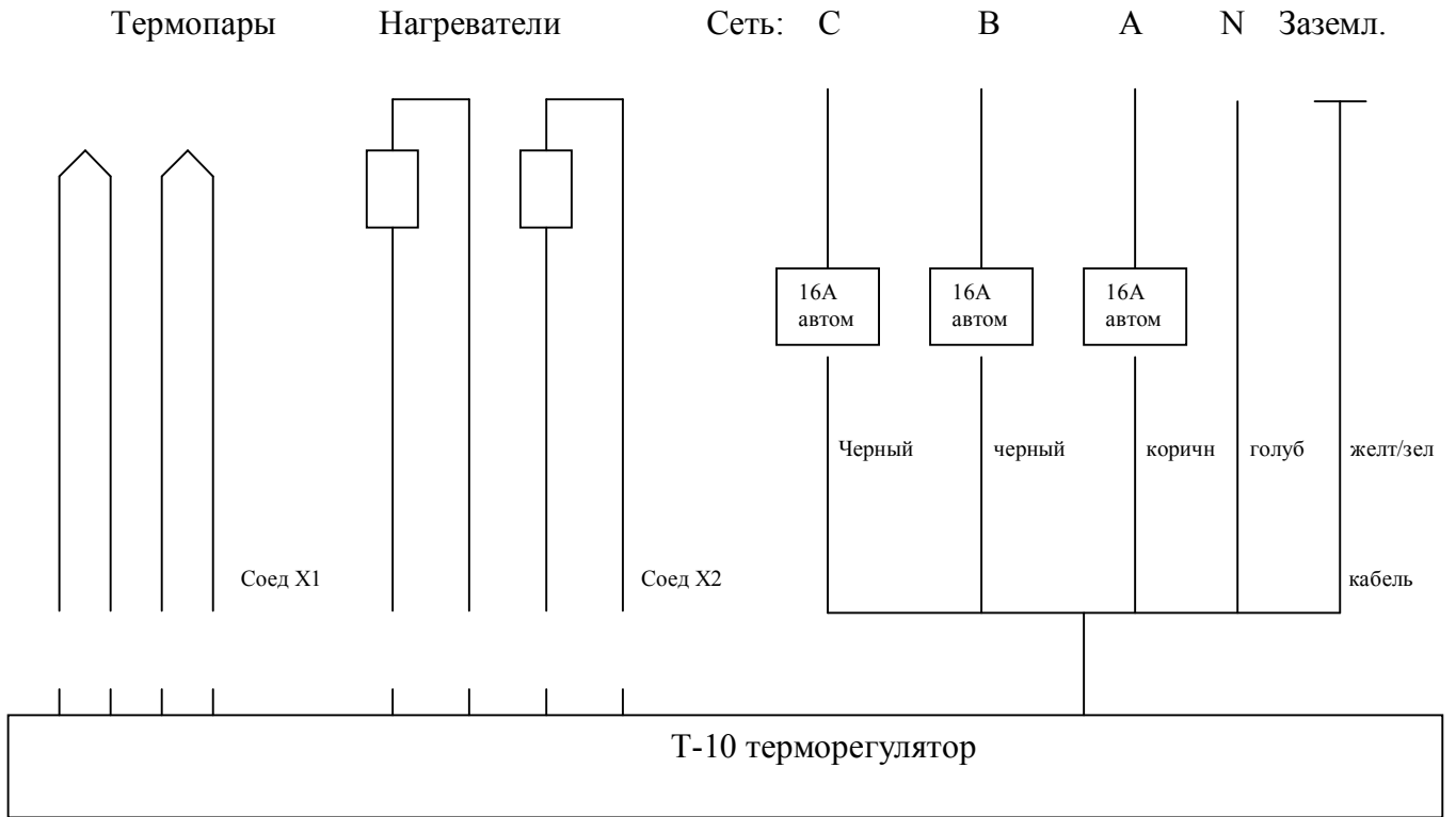
Схема подключения терморегулятора Т-10 к сети питания.
